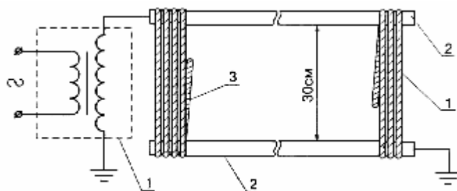
Рис. 2.5. Схема электрических испытаний изолирующего каната 1 - источник испытательного напряжения; 2 - металлическая труба; 3 - испытуемый изолирующий канат
