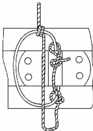
Рис. 2.7. Узел крепления страховочного каната к кольцу
