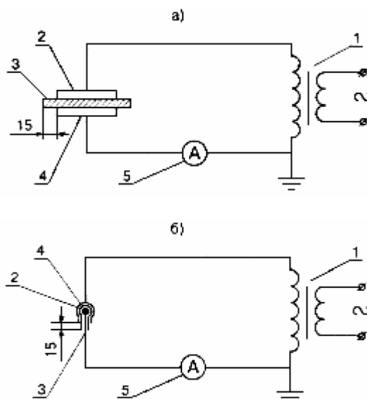
Рис. 2.6. Схемы электрических испытаний гибкого изолирующего покрытия (а) и гибкой изолирующей накладки (б)
