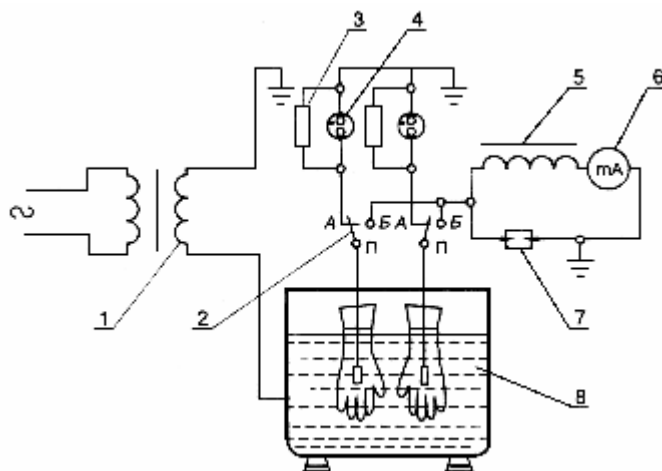
Рис. 2.4. Принципиальная схема испытания диэлектрических перчаток, бот и галош
