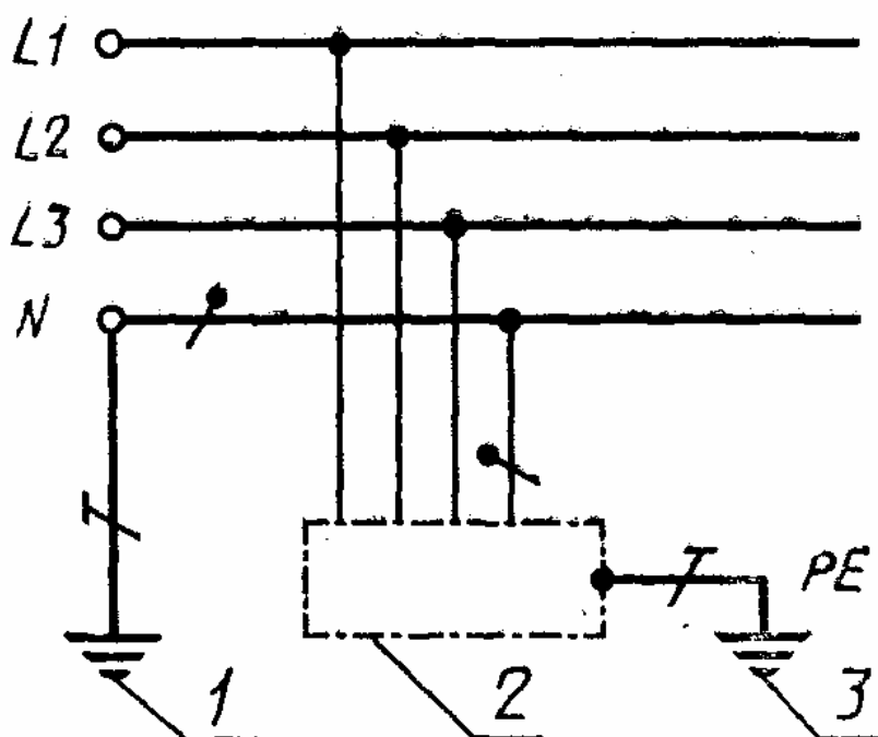
Рисунок 31С - Система TN-C (нулевой рабочий и нулевой защитный проводники объединены по всей сети)
