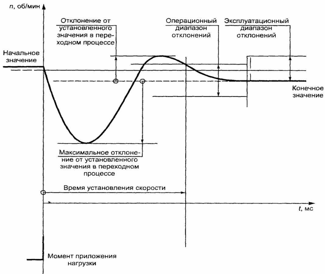
Рисунок А.3 - Временная характеристика при ступенчатом повышении нагрузки и постоянном заданном входном сигнале
