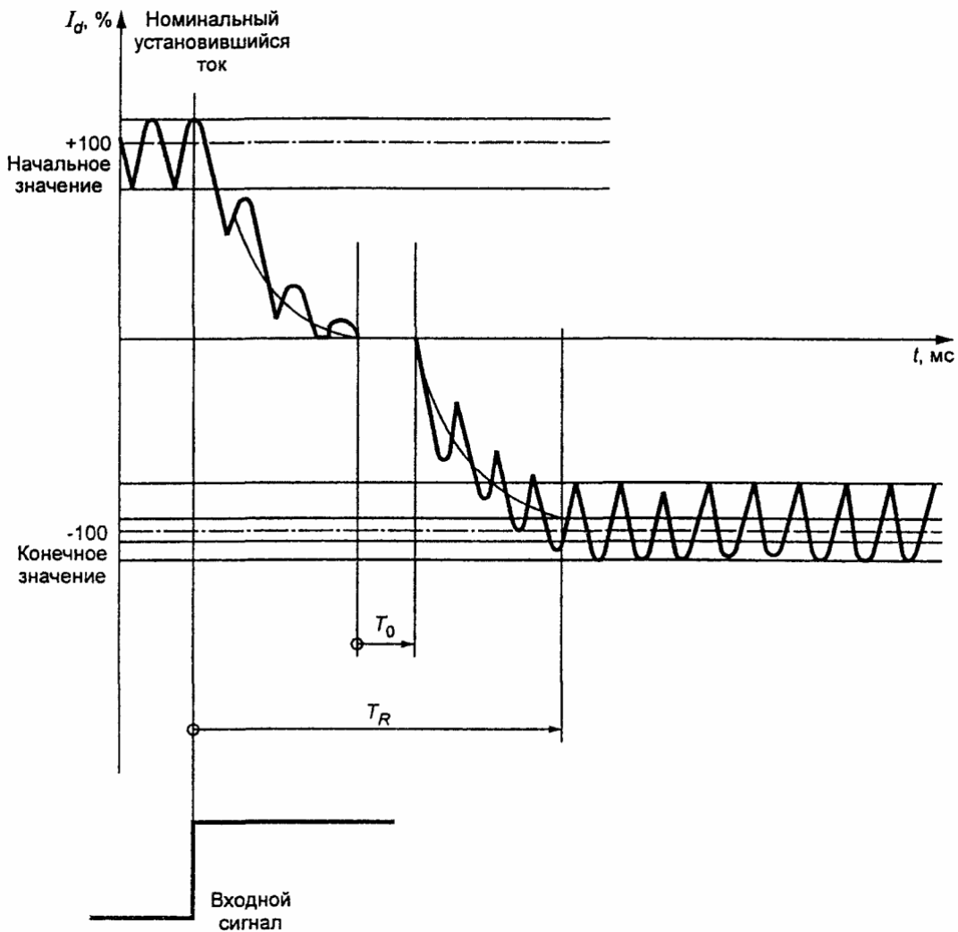
Рисунок А.1 - Диапазон допустимых отклонений
