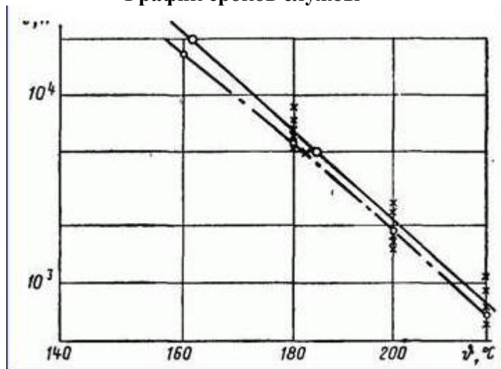
График сроков службы
