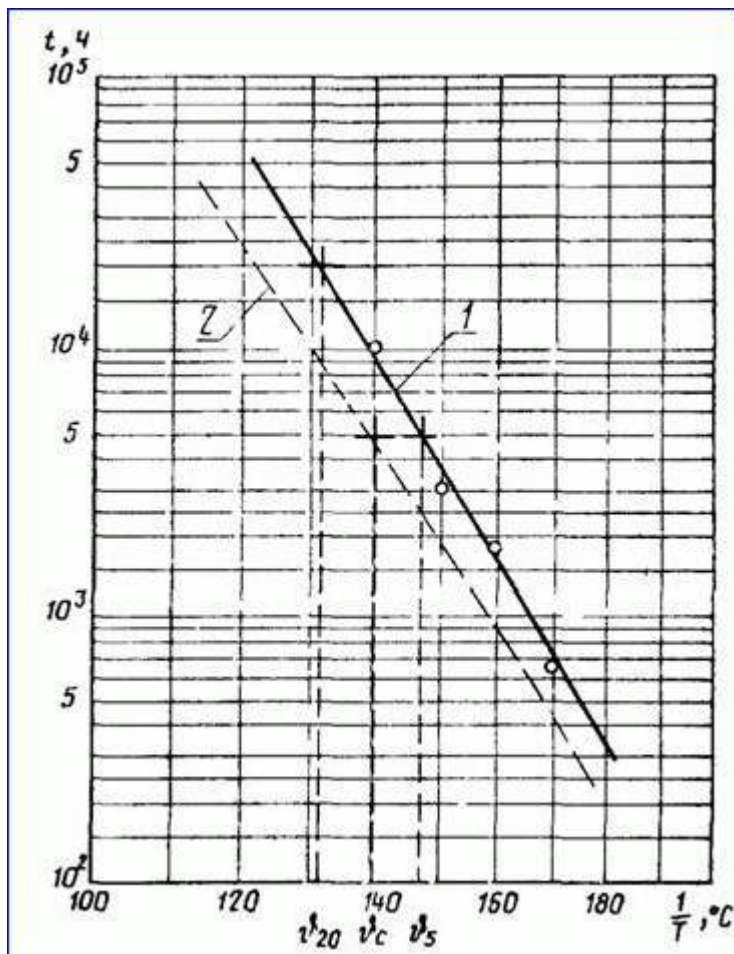
График срока службы эмали-провода
