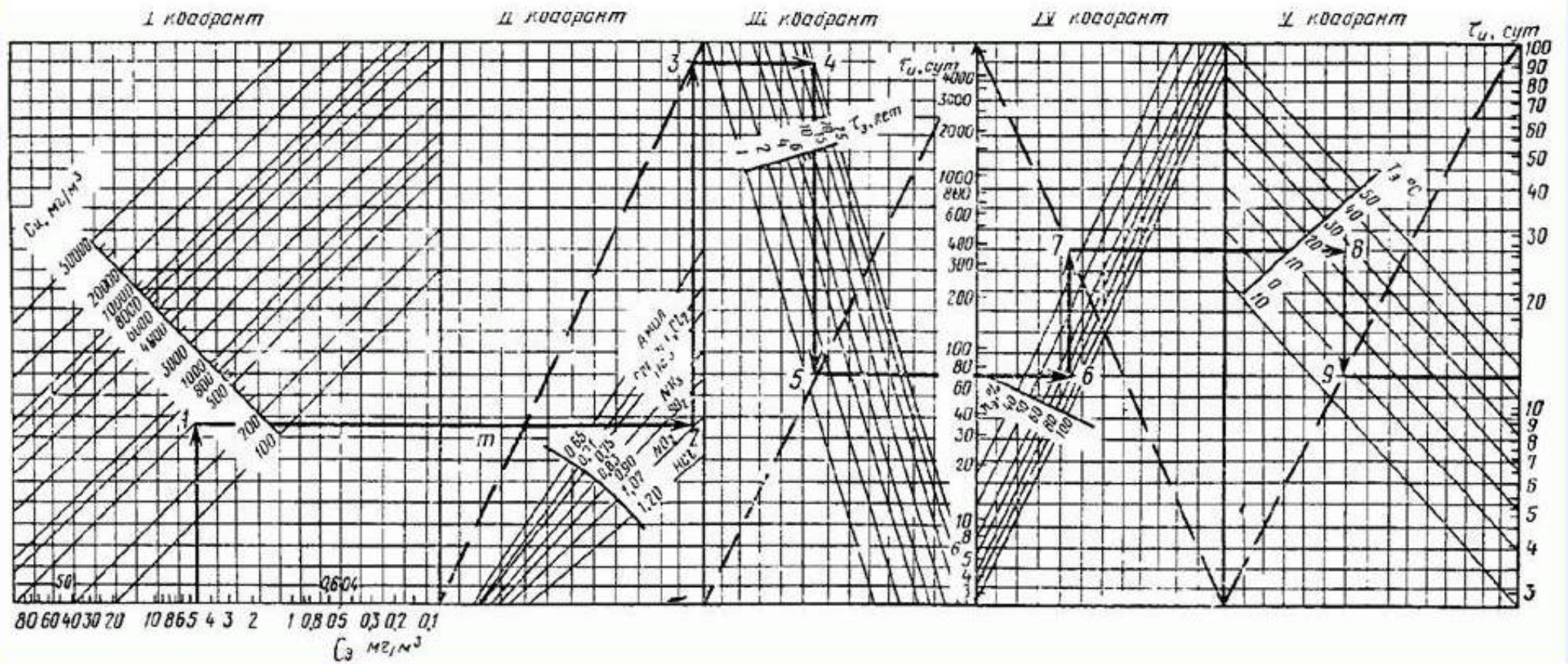
Номограмма определения времени испытаний изделия для заданного времени воздействия среды
