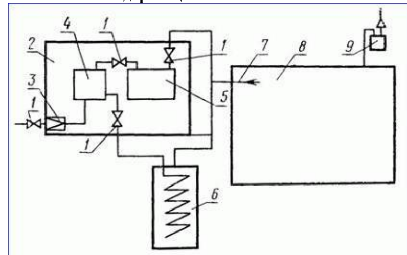
1-двухходовой вентиль; 2-камера испарителя; 3-редуктор; 4 -рессивер; 5-емкость испарителя; 6 -увлажнитель воздуха; 7-форсунка; 8-испарительная камера; 9-электровентиль
