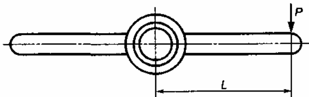
Рисунок 1 — Схема измерения момента вращения
