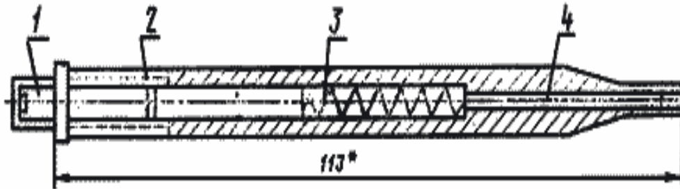
Динамометр для проверки прочности сварки бокового токового ввода
