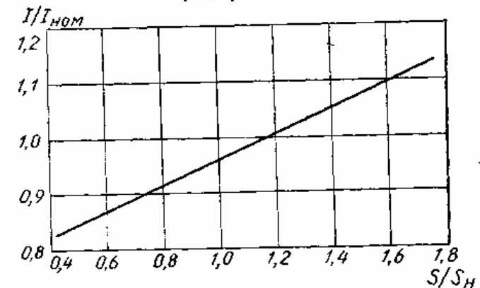
Зависимость тока предохранителя от сечения кабеля
