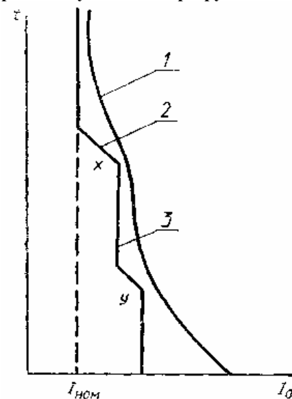
Пример изображения условной перегрузочной характеристики
