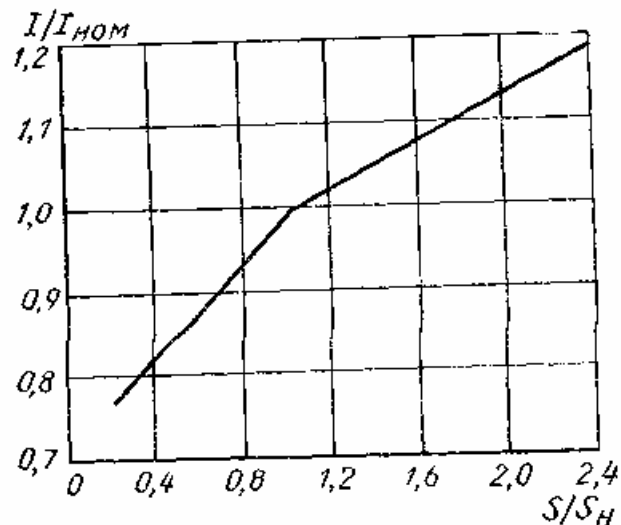
Зависимость тока предохранителя от сечения шины
