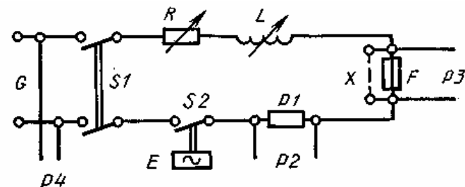
Типовая схема цепи для испытания предохранителя на отключающую способность
