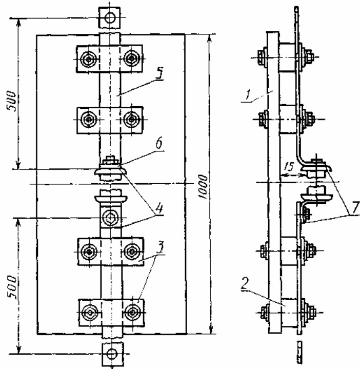
1 — изоляционное основание; 2 — изолятор; 3 — изолированные скобы; 4 — луженая контактная поверхность; 5 — матовая поверхность черного цвета; 6 — место установки термопар; 7 — точки измерения напряжения.
